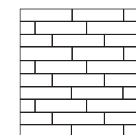
TRAPSGEWIJSVERBAND
