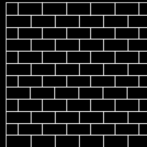
HALFSTEENSVERBAND
